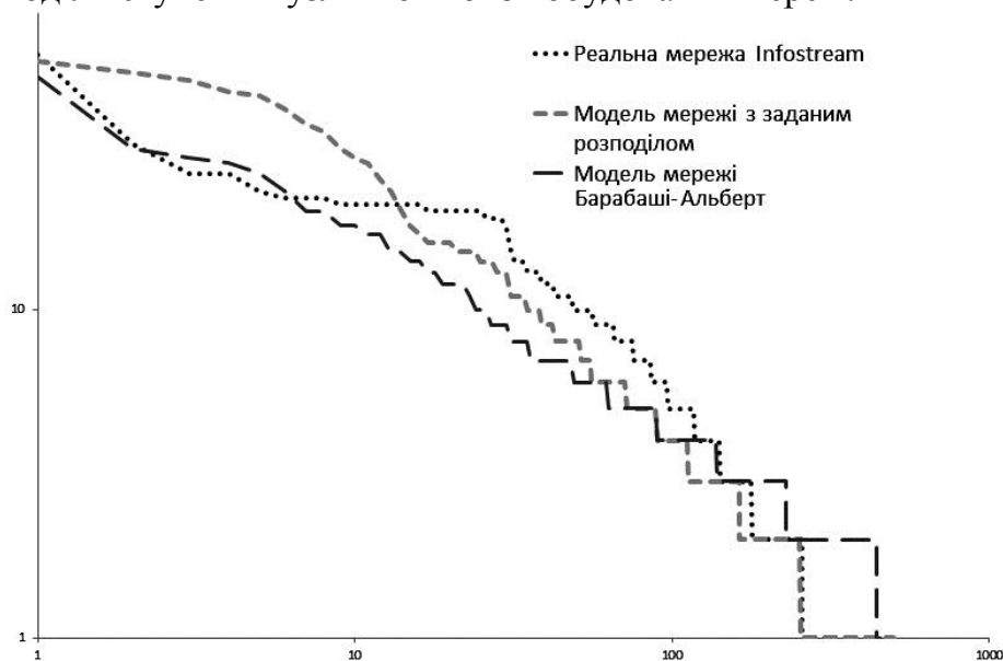
Рис. 4 – Розподіли ступенів мереж, що досліджуються
